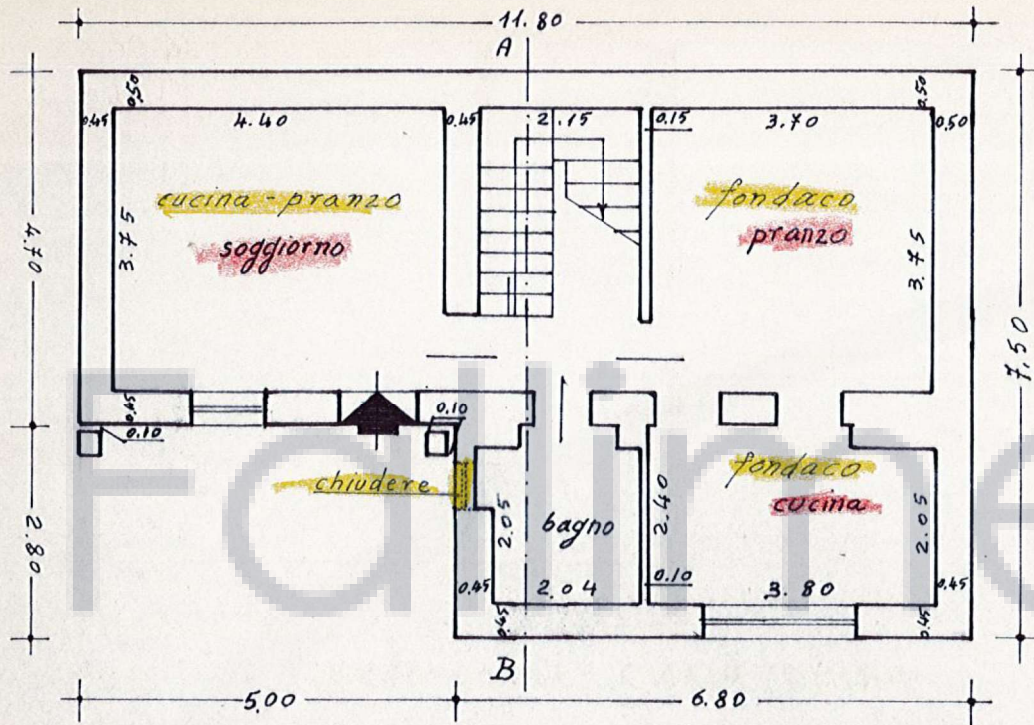
PIANO SOTTOSTRADA
