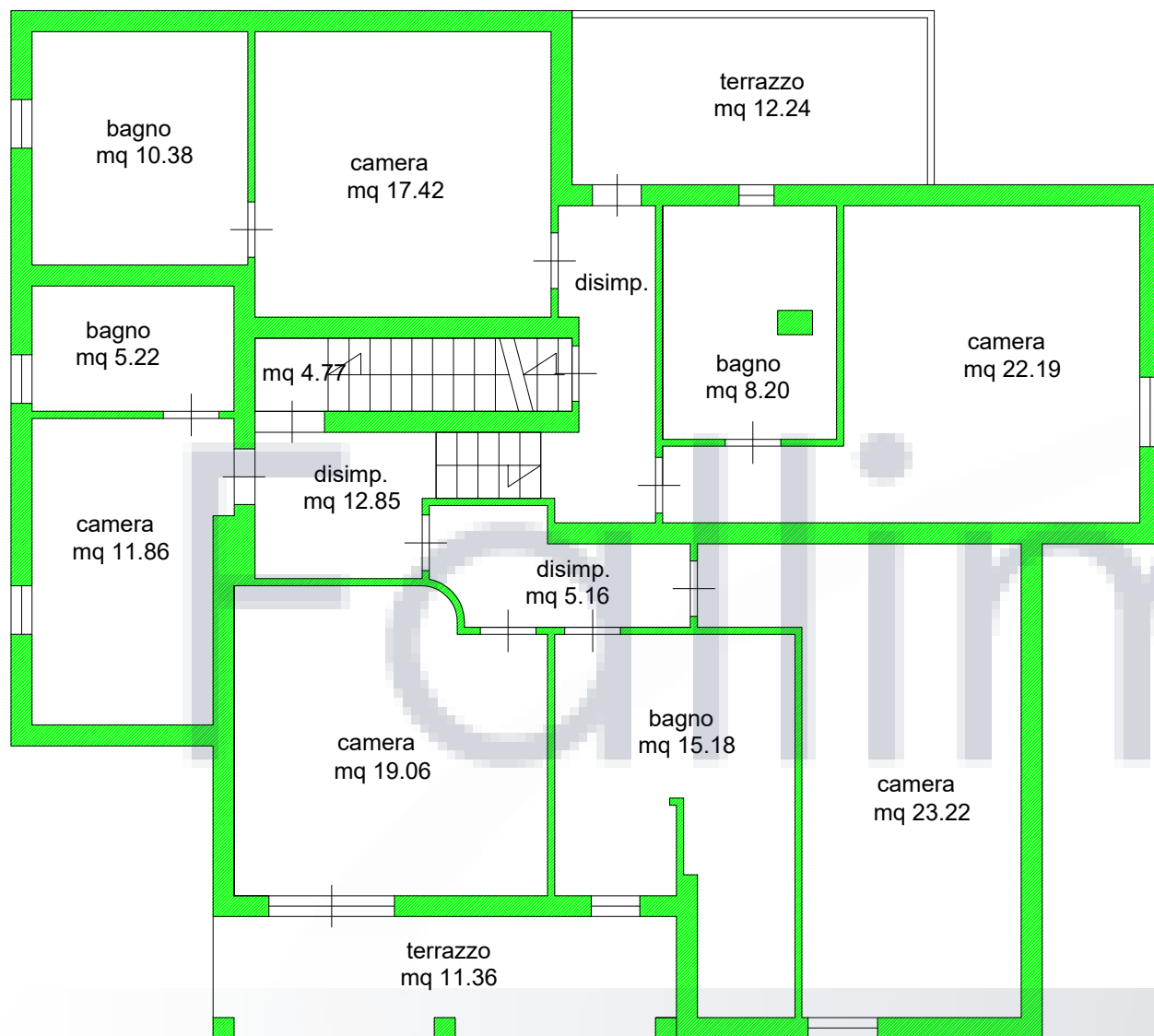
PIANO PRIMO
