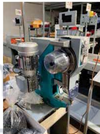
OCCHIELLATRICE
